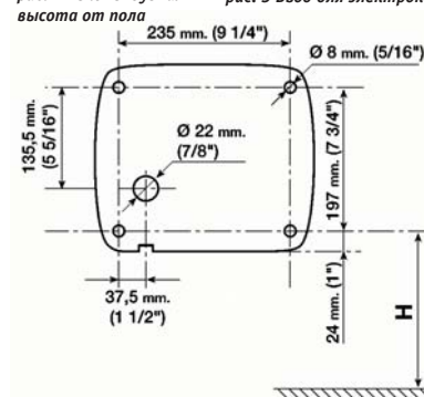
рис. 7 Монтажный шаблон
