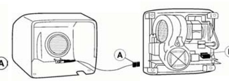
рис. 6 Подключение инфракрасного датчика
