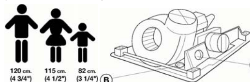
рис. 4 Рекомендуемая высота от пола
