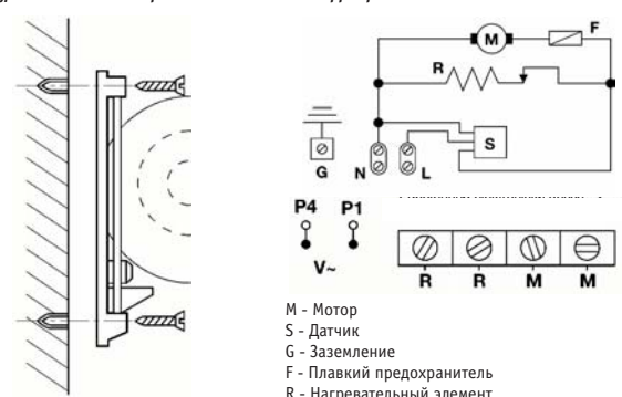
рис. 8 Монтаж сушилки на стену
